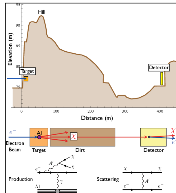
SLAC E137 (1988) Batell, Essig, Surujon (2014)
